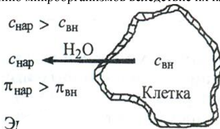
Рис. 3.6. Экзоосмос
